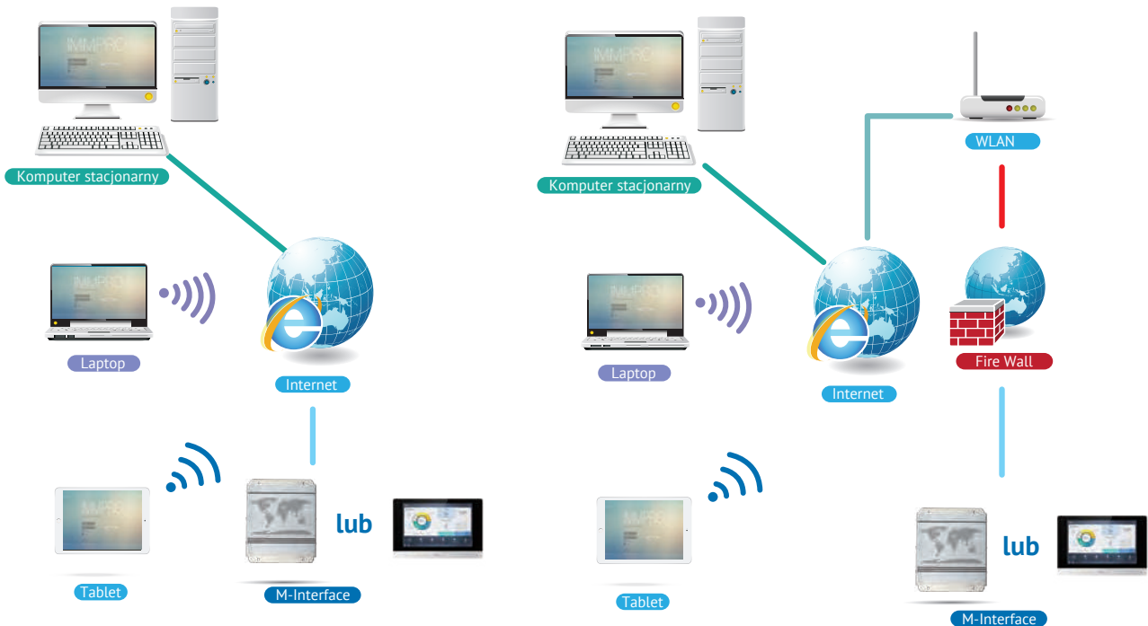
Sieć LAN
